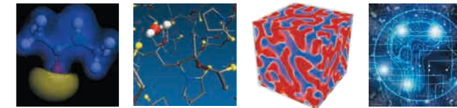
量子化学 Quantum chemistry 分子動力学 Molecular dynamics 粗視化動力学 Coarse-grained dynamics AI・データ科学 AI and data-driven science
