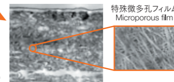
熱交換素子 Heat exchange element
