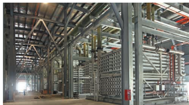
Changi NEWater Plant 規模世界2位、東レのRO膜エレメントを用いた東アジア最大の下水再利用プラント Photo: Sembcorp NEWater Plant, Singapore The world's second largest and East Asia's largest wastewater treatment plant, using Toray RO membrane elements.
